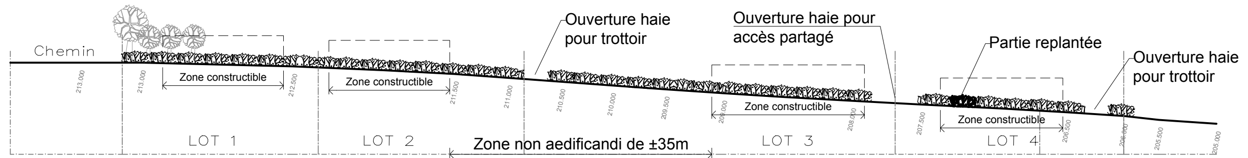
COUPE AA' (Urbanisation) (Front de voirie - Haie)
