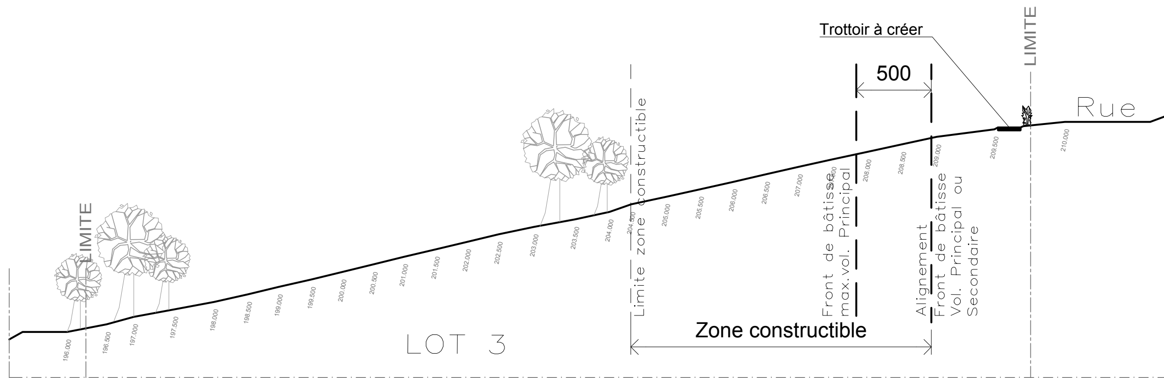
COUPE BB' (Urbanisation)
